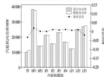
图8 额定工况汽轮机各模块功率模拟误差分析
