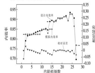
图7 额定工况汽轮机内效率模拟误差分析
