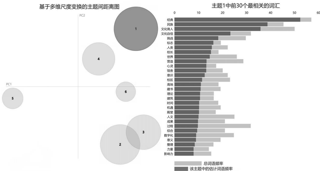
图 2 使用 pyLDAvis 模块输出的可视化主题聚类结果 ①
